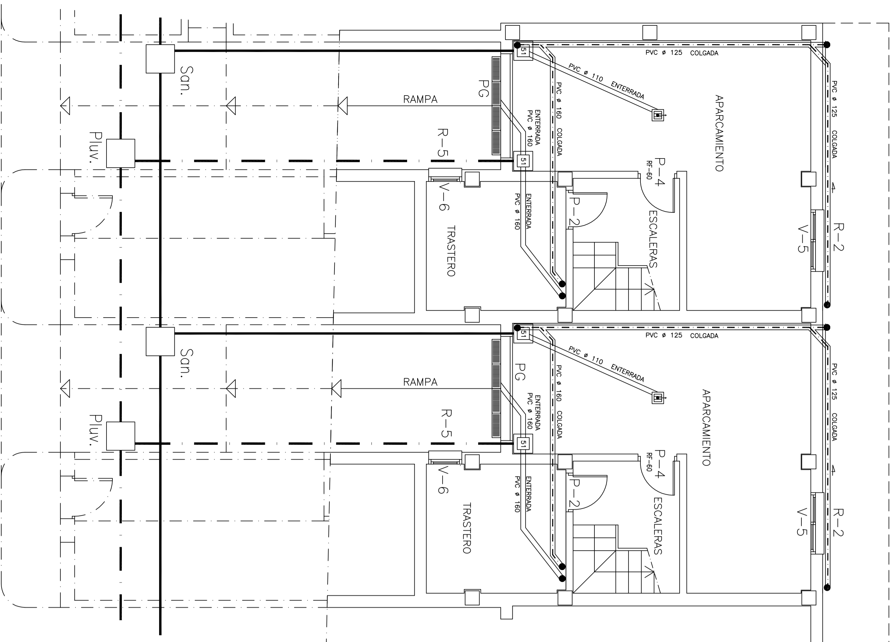
PLANTA SEMISOTANO
