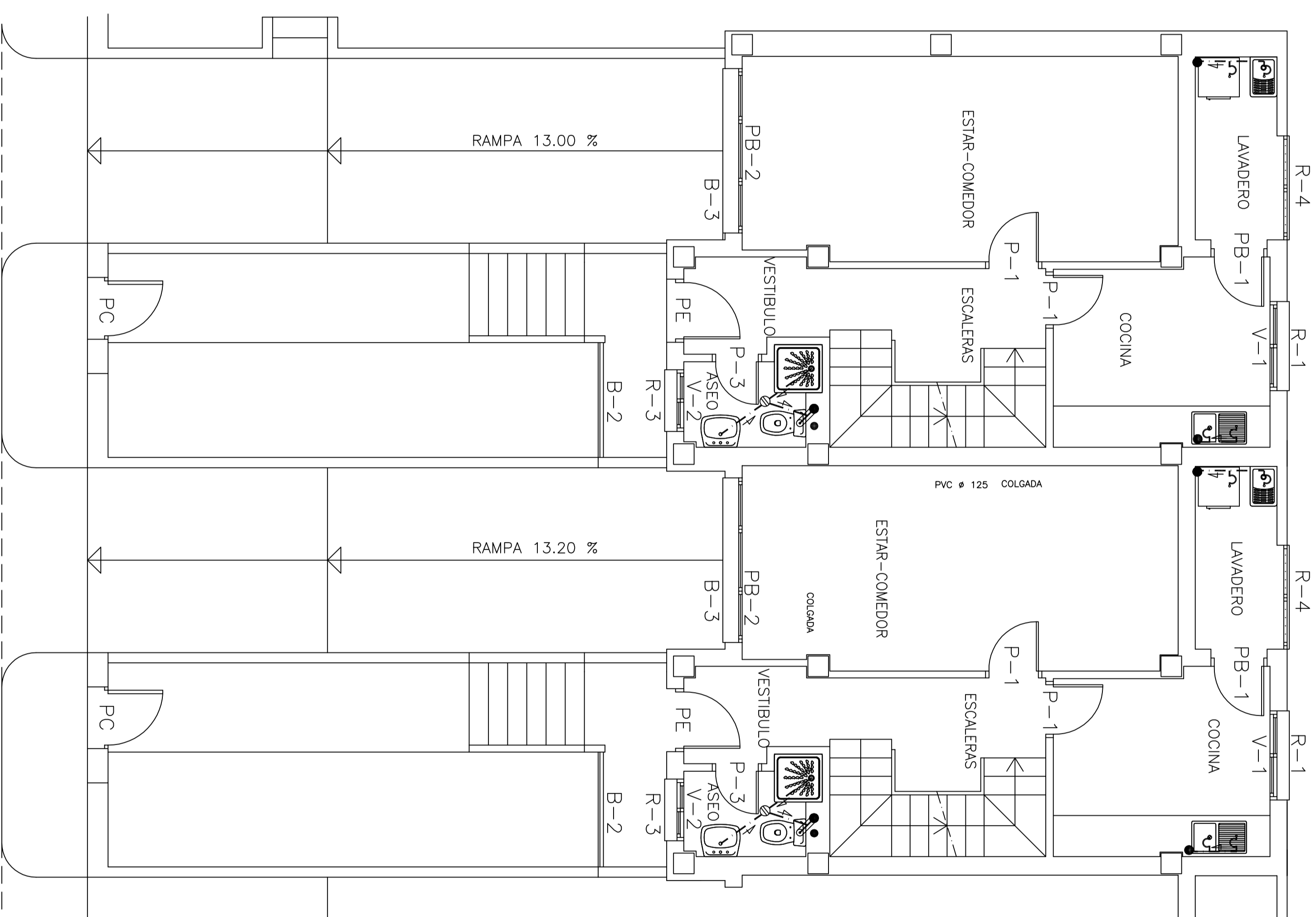
PLANTA BAJA
