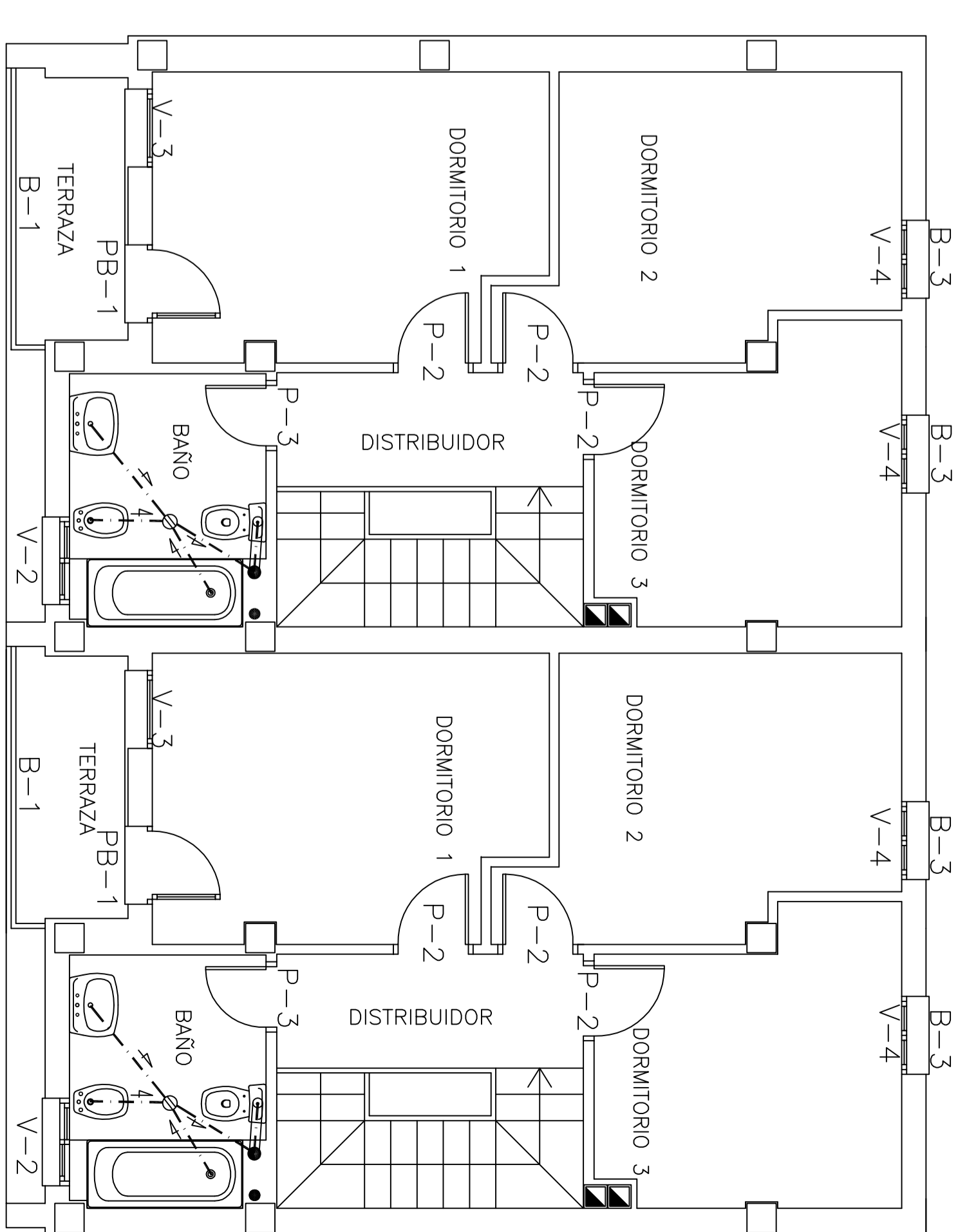
PLANTA ALTA
