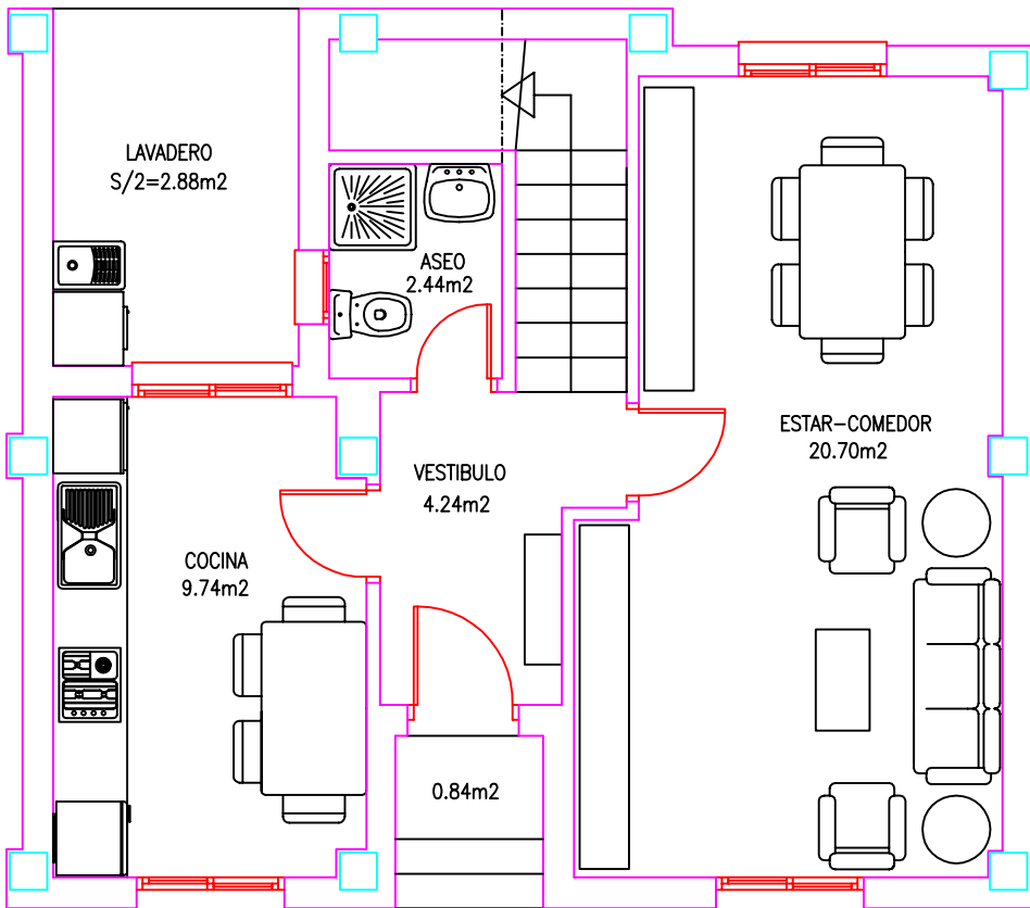
PLANTA BAJA
