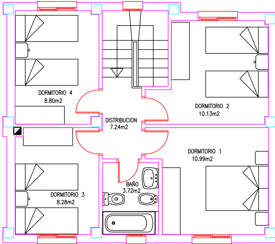
PLANTA ALTA
