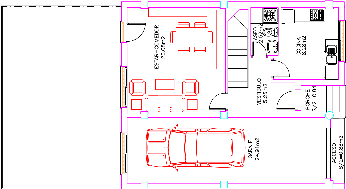
PLANTA BAJA
