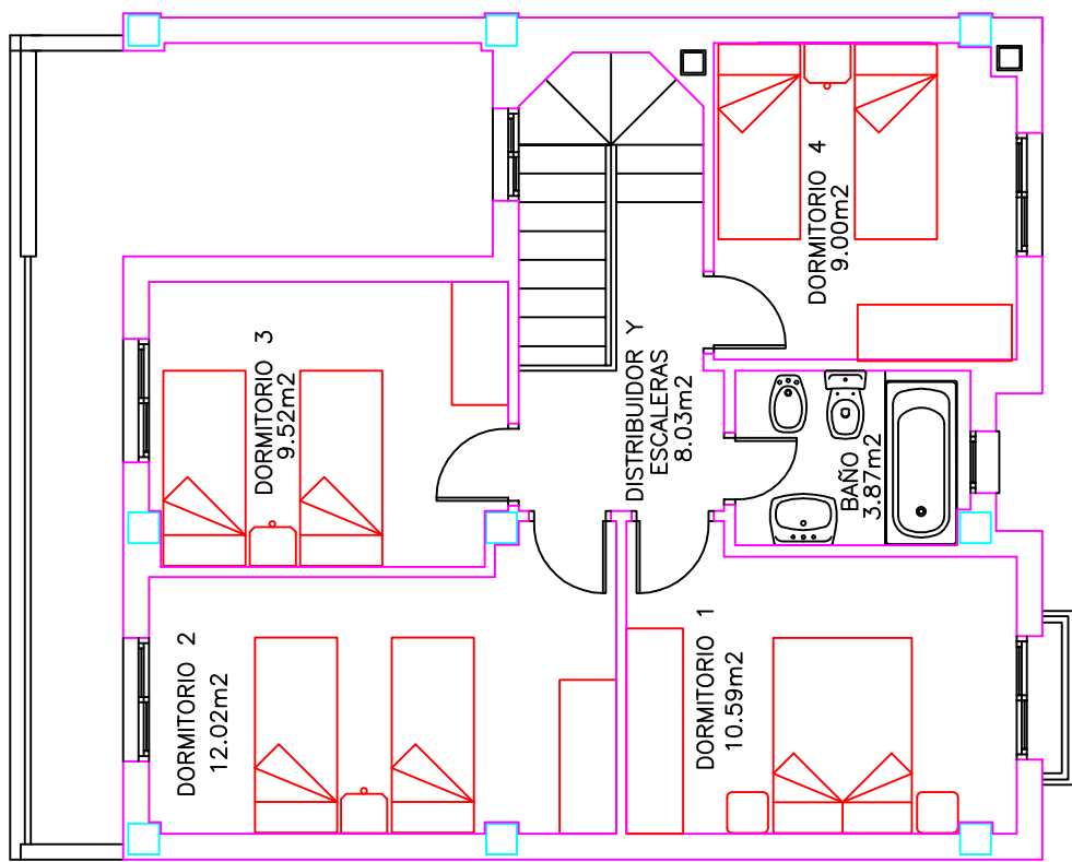
PLANTA ALTA
